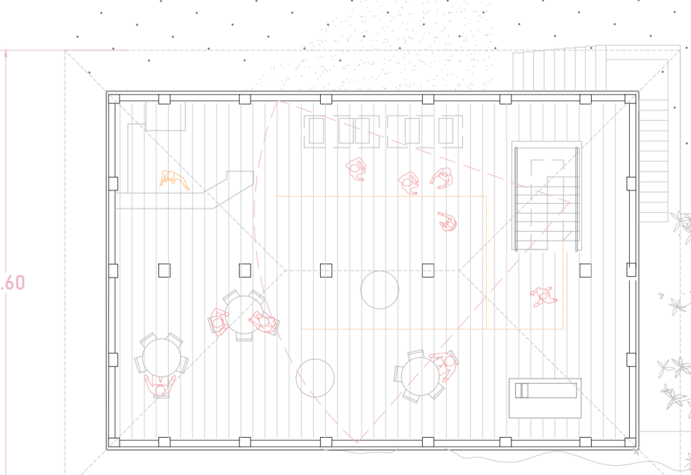
PLANTA_03
