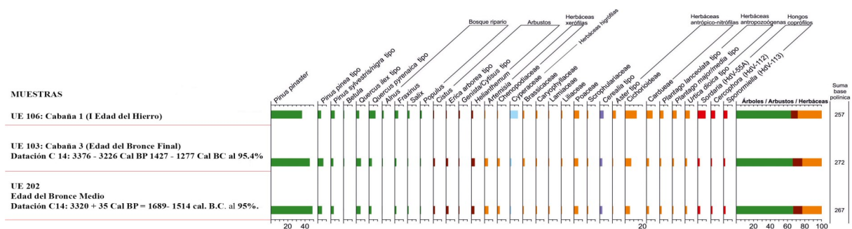
LAM. 7. Histograma polínico del yacimiento de La Peña del Moro.
