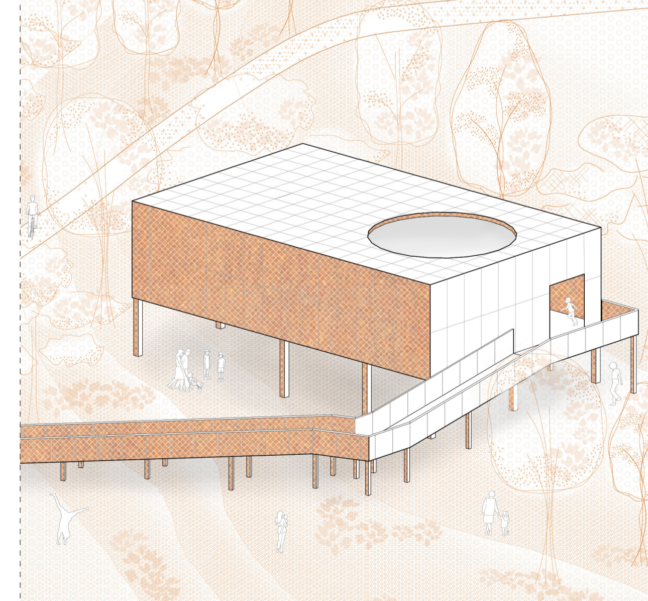
ISOMETRÍA
