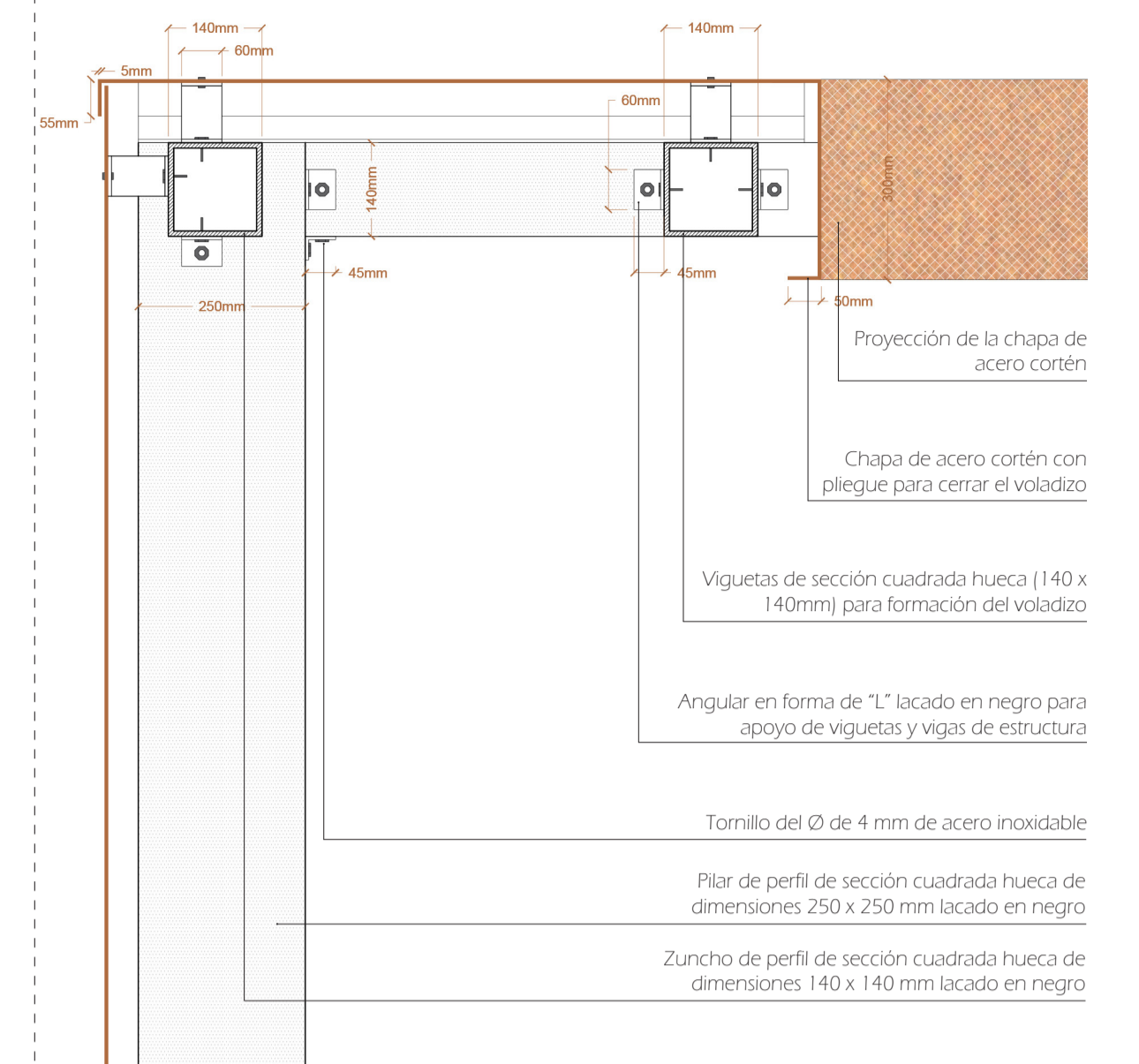
DETALLE 1 SECCIÓN DEL VOLADIZO
