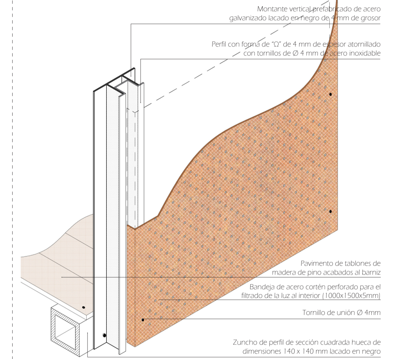
DETALLE 2 SECCIÓN DEL RECURRIMIENTO EN FACHADA
