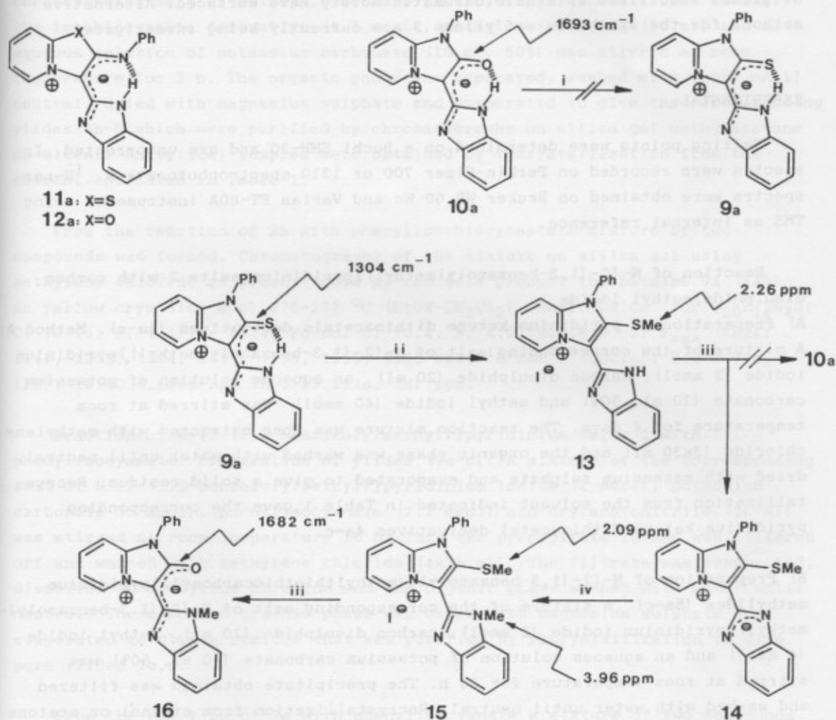
Scheme 5.1, Lawesson's reagent, \text{CH}_2\text{Cl}_2 -toluene, reflux. ii, EtOAc/MeI, r.t.; iii, MeOH/NaOH (aq., 50%), r.t.; iv, EtOAc/MeI, r.t.
