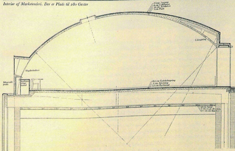
Snit Vilhelm Lauritzen: Statsradionens Bygning. Markendeti, Interior og Snit 1:100. I højre Side er Tagets Friliggende 25 m. Overdelen af Stutte 2 ses som den nederste Æske med Loft af Træ, belastet med Sand 137
