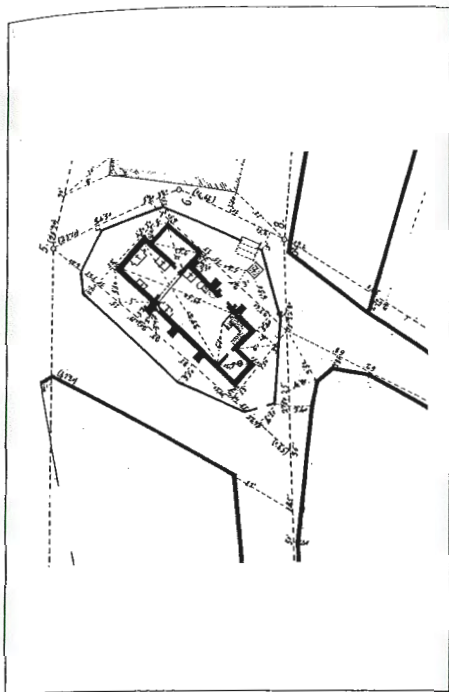
Iglesia parroquial de San Pedro Advíncula. Planta, 1869. IGN
