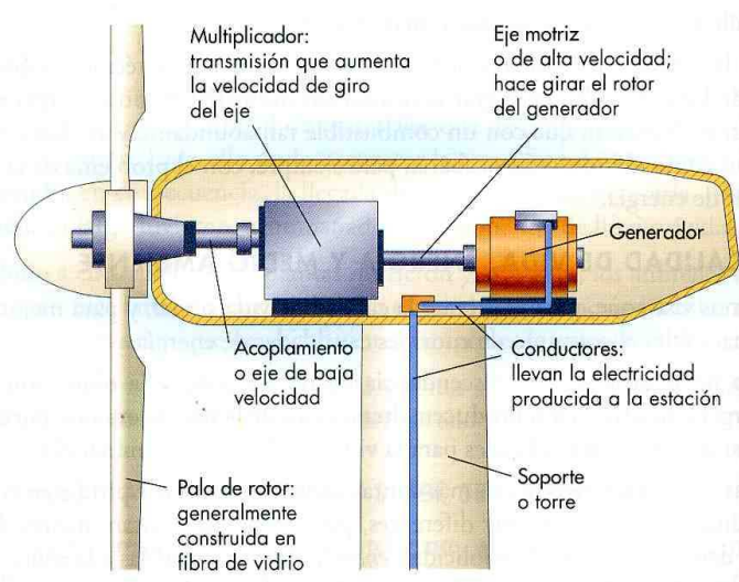
Figura 1. Esquema del funcionamiento de un aerogenerador
