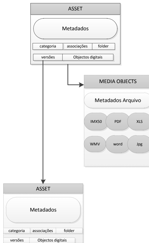
Figura 63 - Modelo de representação de um Asset em ARKEMEDIA
