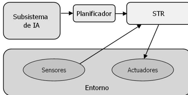
Fig. 1. Esquema de una arquitectura cooperativa para un sistema de inteligencia artificial en tiempo real
